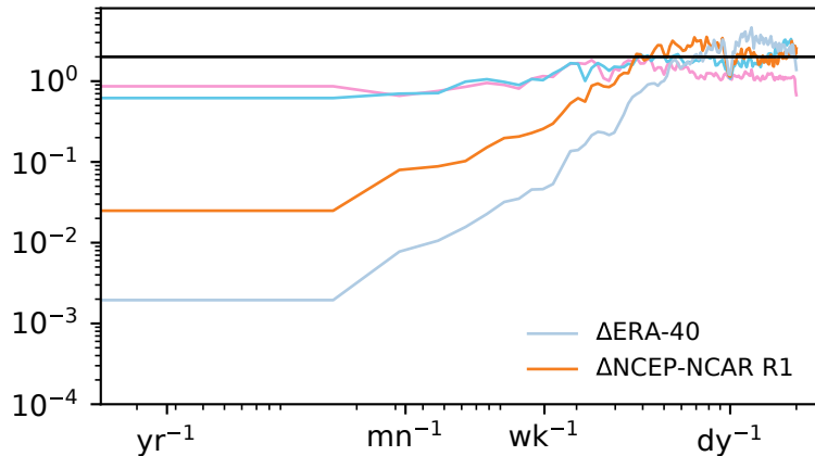
(d) u 500 hPa, 40° N 1958 to 1978
