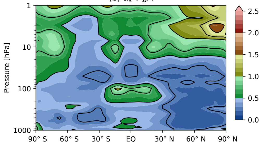
(d) \alpha_r T JJA
